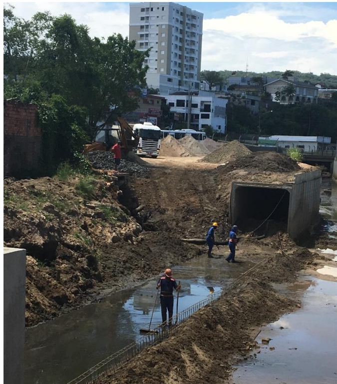
Figura 8: Trabalhadores realizando o preparo da base. (Fonte: Dos Autores 2019)
