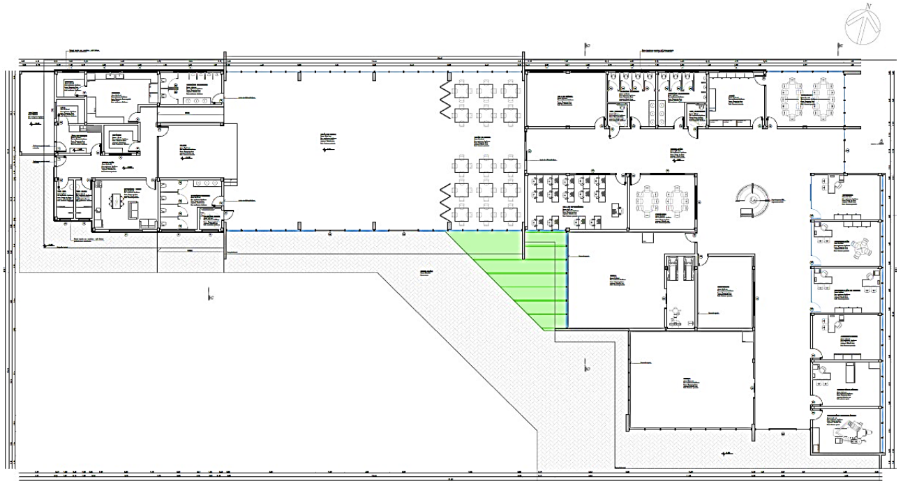
Figura 2: Planta Baixa do Centro do Idoso. (Fonte: Autores 2020).
